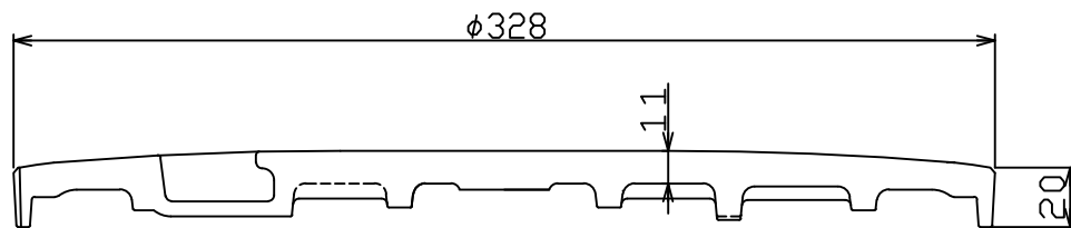
A-A' 断面図
